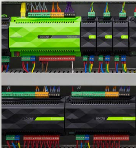
Die Installation des Miniservers (grün) und ergänzender Module.
